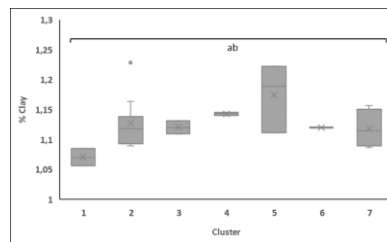
(o) % Clay
