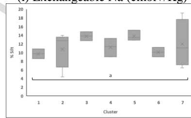
(l) % Silt
