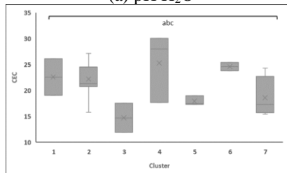
(d) CEC
